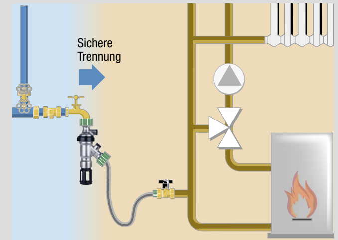
Normgerechter Anschluss beim Nachfüllen der Heizungsanlage.
