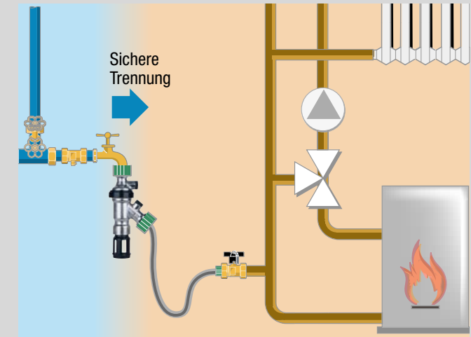
Normgerechter Anschluss beim Nachfüllen der Heizungsanlage.
